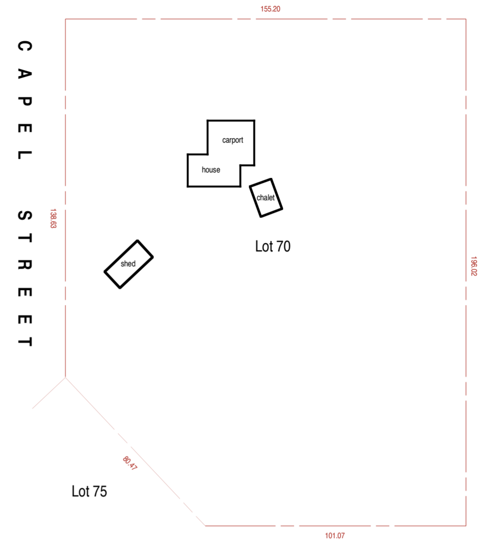
SITE PLAN (1:1000)
